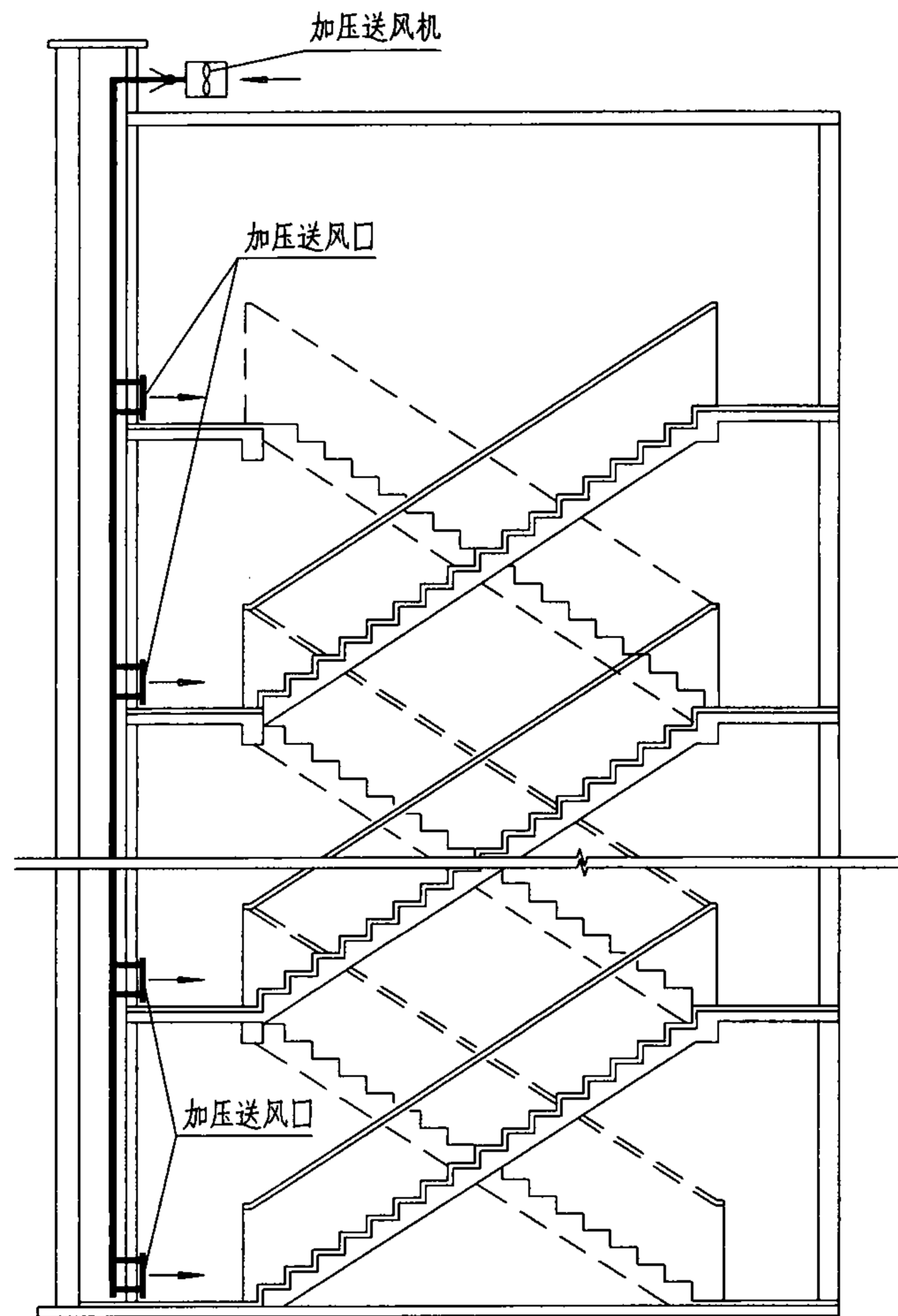
A-A剖面图
