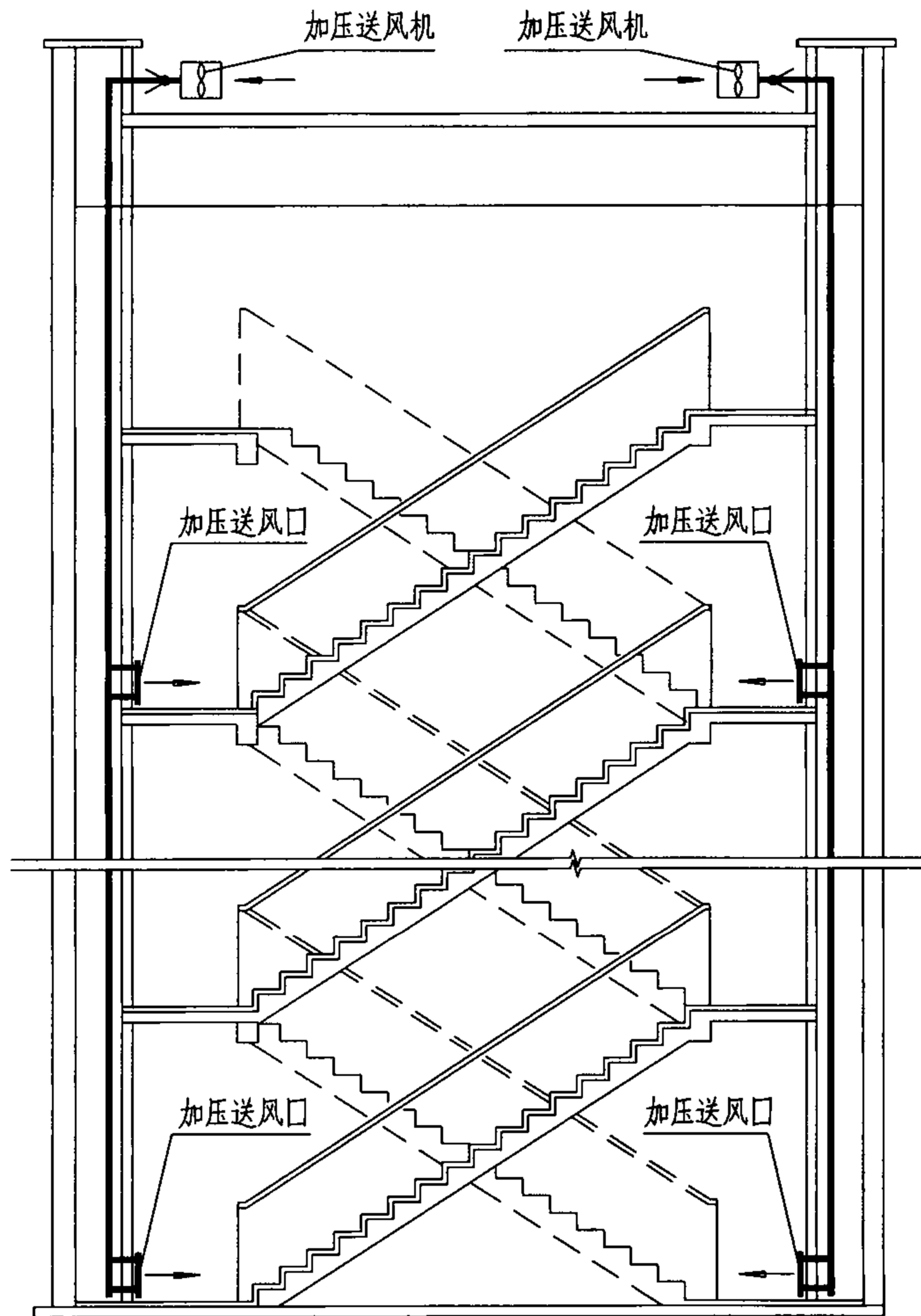
A-A剖面图
