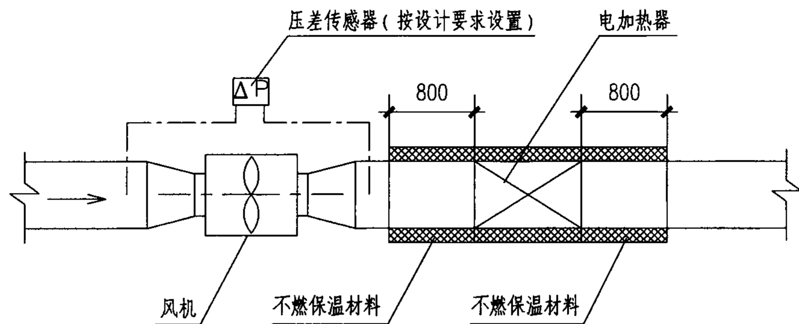
电加热器安装示意图
